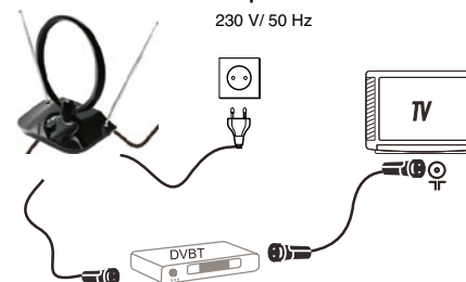
(Рис. 2) Прямое подключение к телевизионной приставке
