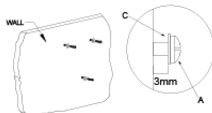
(B) 8x40 Пластиковый дюбель (3)
