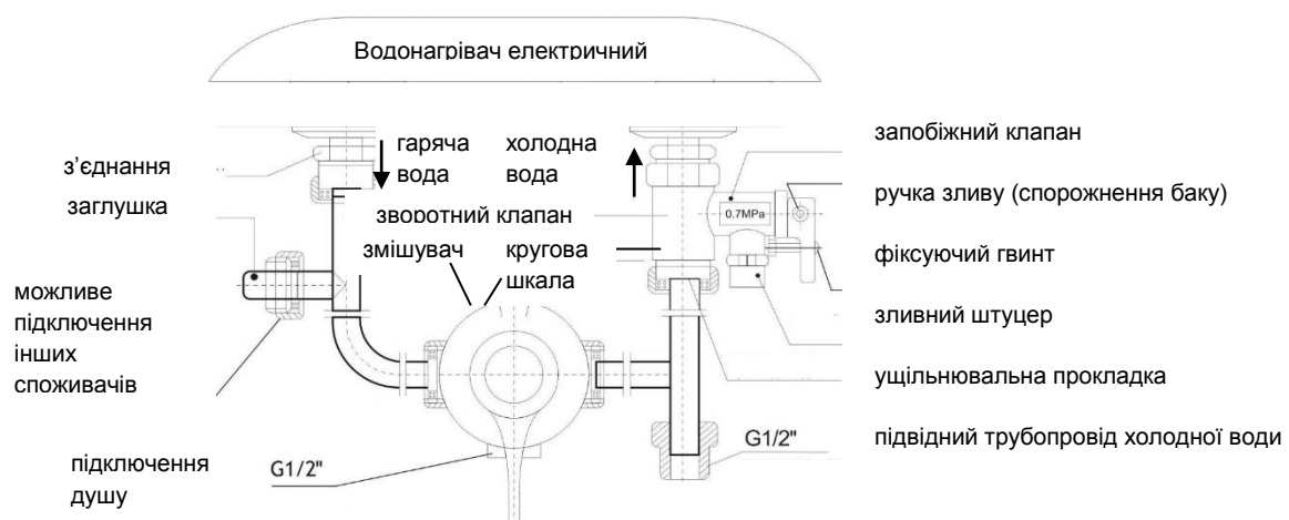
Схема підключення
