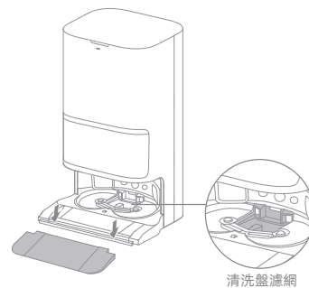
清洗盤濾網
