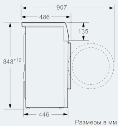
Размерные чертежи
