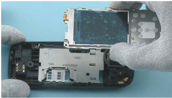
13) Remove the ENGINE MODULE.
