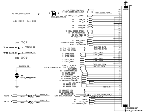
MS/SD DB CONN. --MB Side
