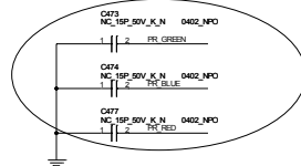
Docking DB CONN. --MB Side
