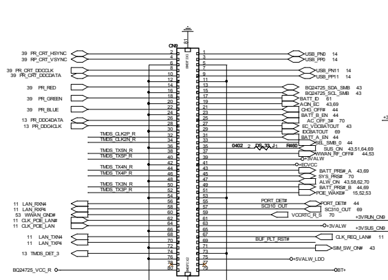
Docking DB CONN. --MB Side
