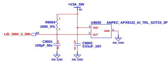
LID Switch
