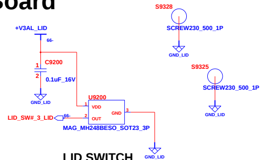
LID SWITCH
