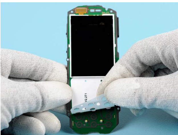
15) Peel back the DOME SHEET.
