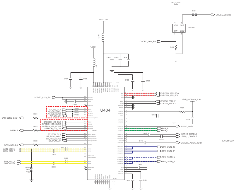
AUDIO CODEC
