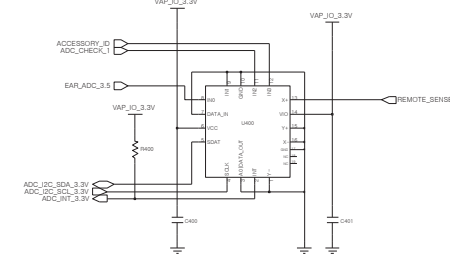
ADC IC
