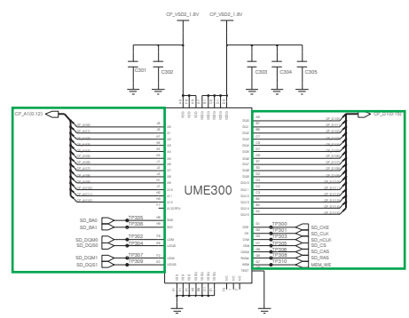
Mobile DDR SDRAM 512Mb(16M x 16)
