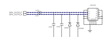
Right SPK / MOT conn
