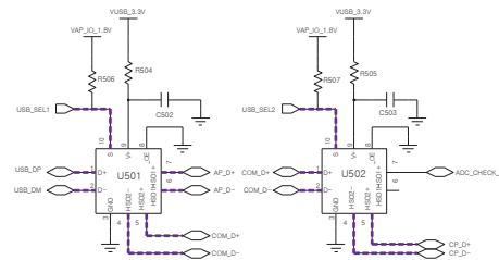
USB SWITCH IC
