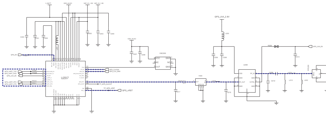
GPS LNA
