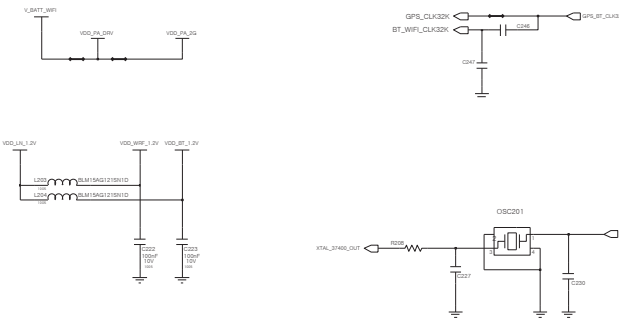
BT/WIFI OSC
