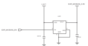
EAR_MICBIAS 2.8V
