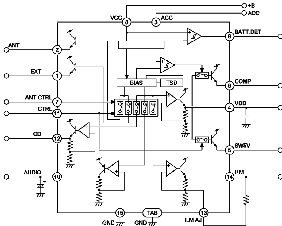
IC701 : C0DAZHF00004
