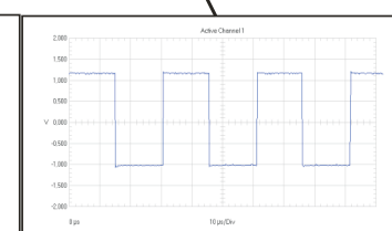
32 kHz SLEEPCLK
