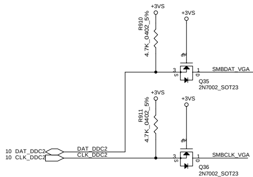
DVI Interface
