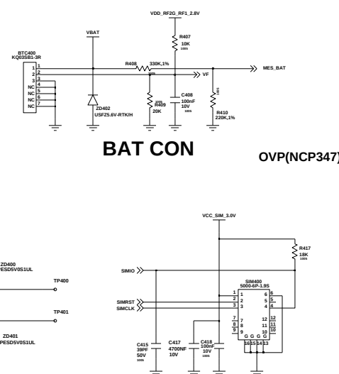
SIM CON
