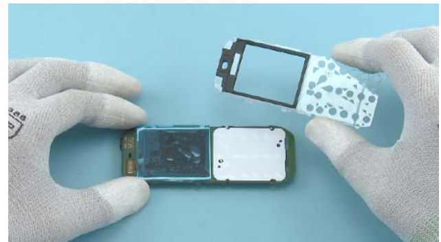
16) Remove the LIGHT GUIDE.
