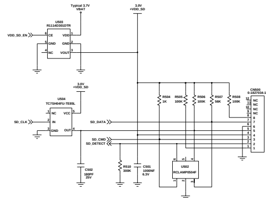
T-FLASH
