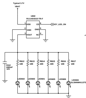
KEY_LED
