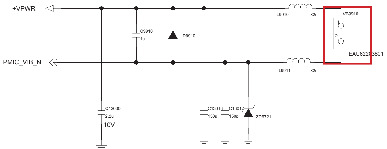
Motor
