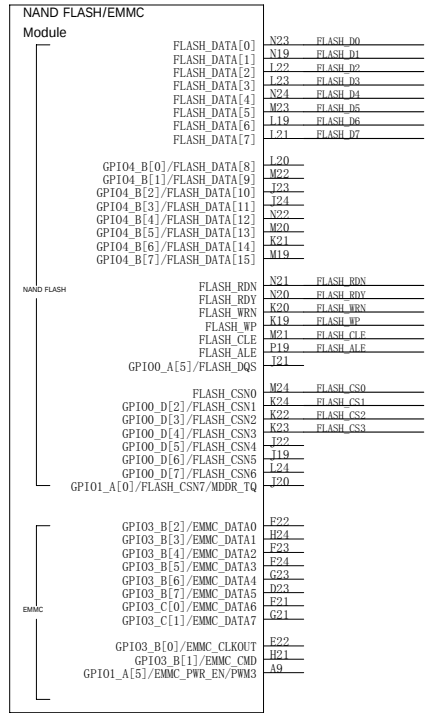
U1-E RK2918 BG512
