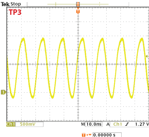
CAM_70MHz PCLK
