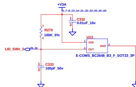
LID SWITCH
