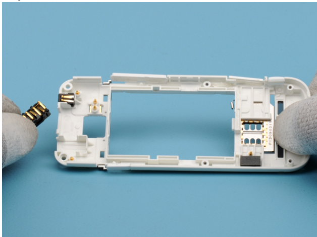
26) Remove the CONN AV 4POL D2.5.
