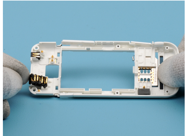
25) Release the CONN AV 4POL D2.5.
