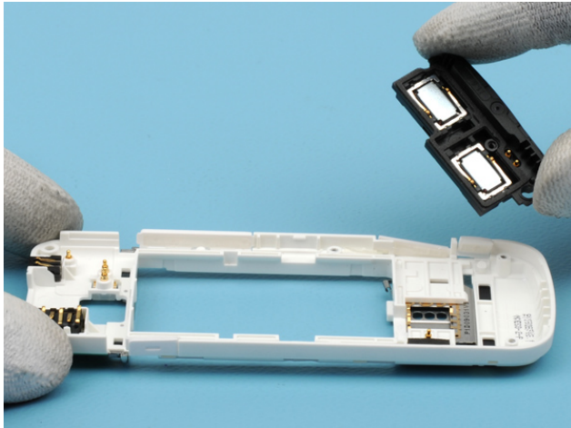
24) Remove the ANTENNA ASSY.
