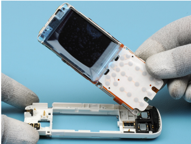
12) Remove the B-COVER.
