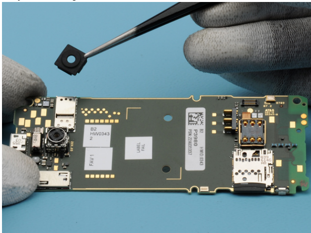
20) Remove the CAMERA BOOT.
