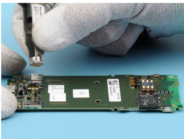
22) Remove the CAMERA.
