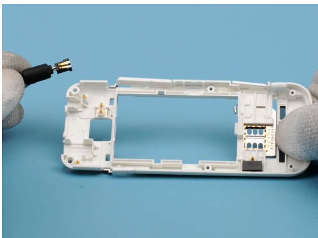
28) Remove the CONN CHR DIA 2.0MM COMPRESS.
