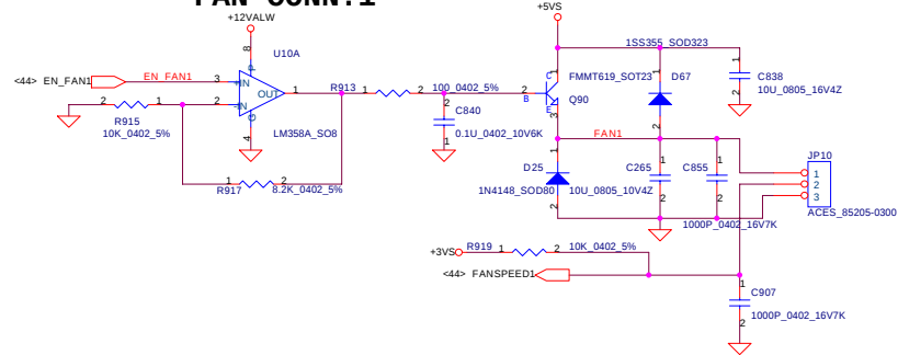
FAN CONN.1
