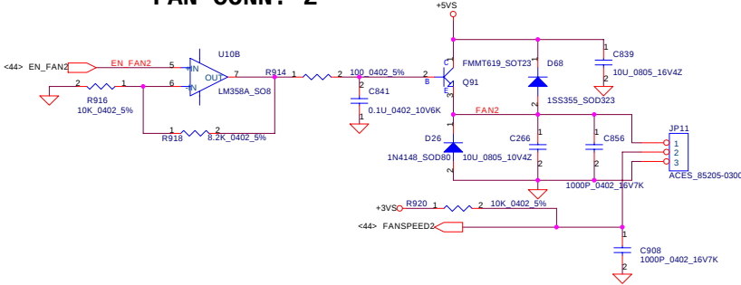
FAN CONN. 2
