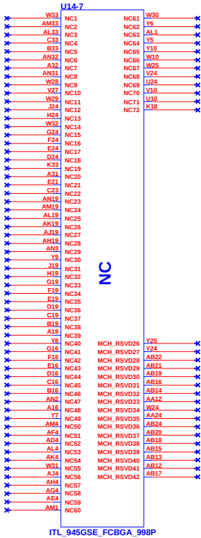
ITL 945GSE_FCBGA_998P
