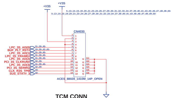
TCM CONN
